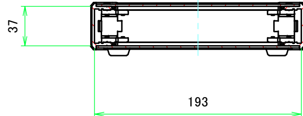
B-B ( 1 : 3.5 )
